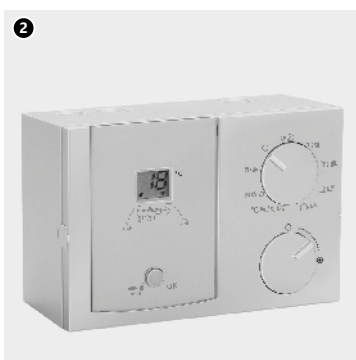
Slika 53. Regulacijski elementi KAN-therm centralnog sistema mješanja (SM4 aktuator (1) regulator vremena(2))
