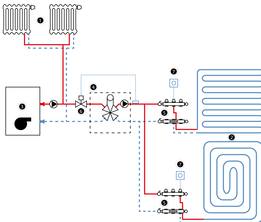
Slika 54. Dijagram centralnog sistema miješanja s poluautomatskom regulacijom
