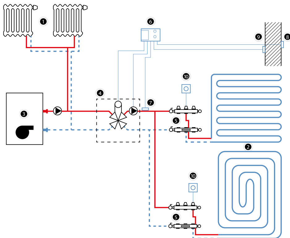
Slika 52. D i j a g r a m centralnog sistema mješanja s automatskom regulacijom
