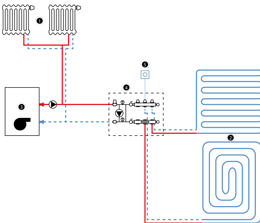
Slika 57. Lokalni sistem miješanja
